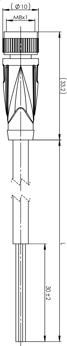
Projektionsansicht
