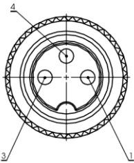
Steckbild
