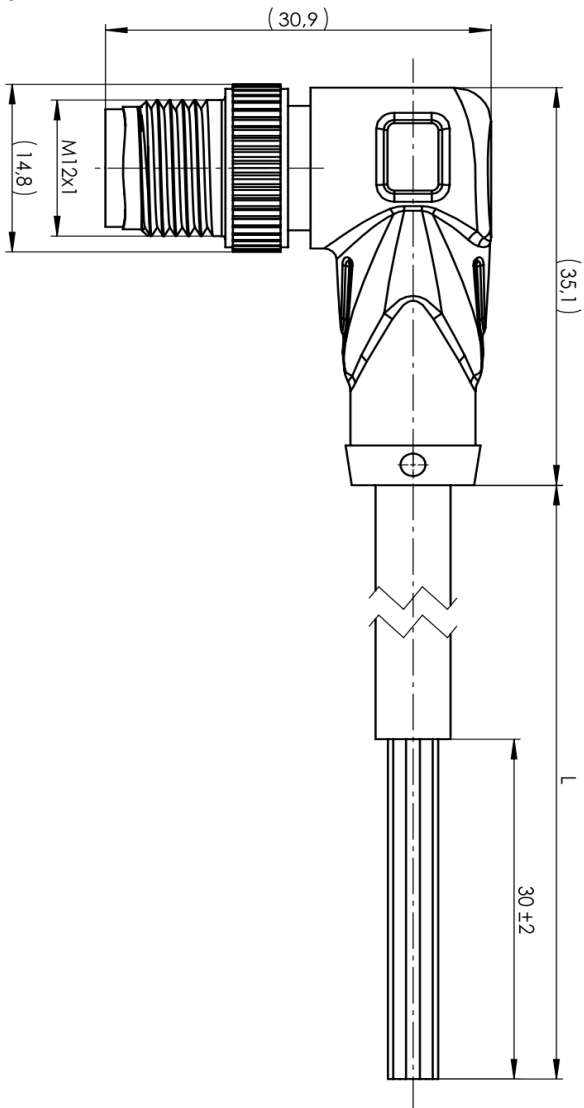
Projektionsansicht
