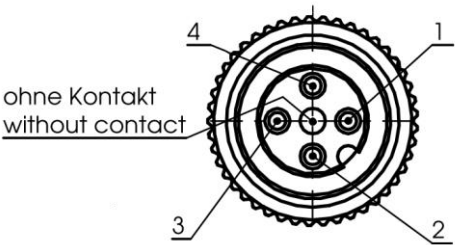
Steckbild
