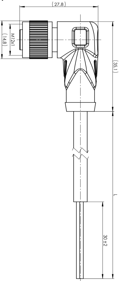
Projektionsansicht
