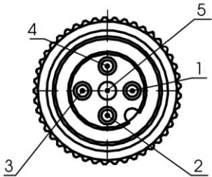
Steckbild
