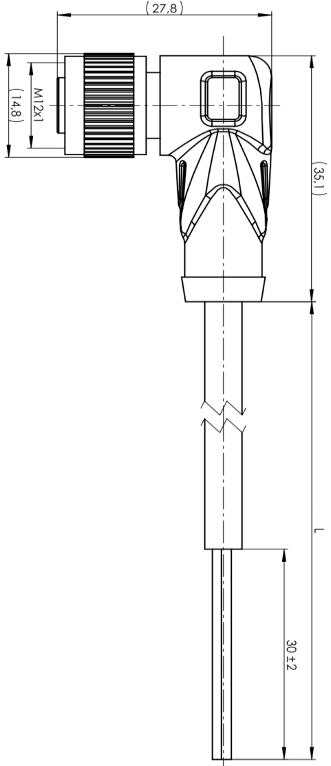
Projektionsansicht
