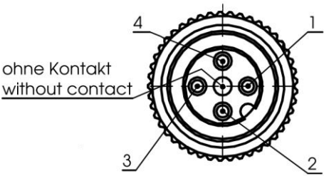
Steckbild
