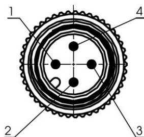
Steckbild
