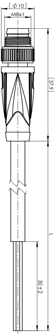
Projektionsansicht
