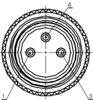
Steckbild
